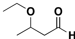
3-ethoxybutanal
