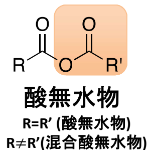
アシル基
