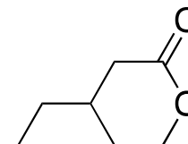
4-ethyloxacyclohexan-2-one
