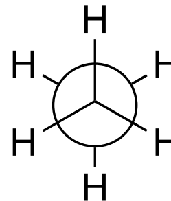
Newman投影図
